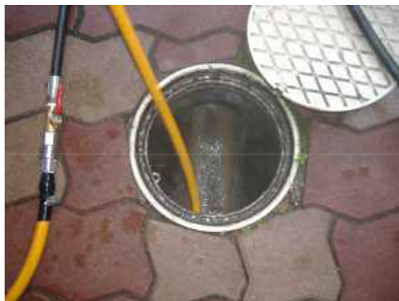
共用部排水管
